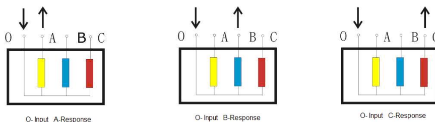
Figure 3 YN Wiring
