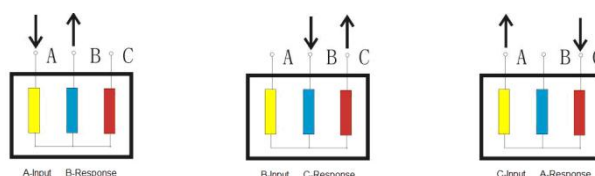
Figure 4 Y Wiring
